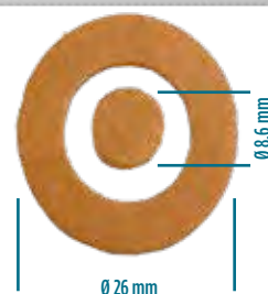
⊕ Pastille détecteur de pluie et lumière pour : VW ancien modèle. Vendue à l'unité REF : PPP-WST61H
