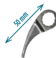
⊕ Lame contre-coudée 50 mm D'autres modèles sur demande. Vendue à l'unité REF : PPP-WST45D
