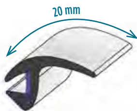
➔ PROFIL UNIVERSEL PVC Profil PB 20 mm avec butyl rouleau 23 m REF : PPP-JT004
