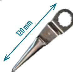
⊕ Lame contre-coudée dentelée 120 mm D'autres modèles sur demande. Vendue à l'unité REF : PPP-WST45X
