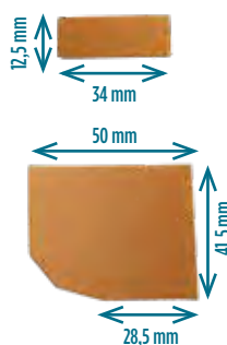
⊕ Pastille détecteur de lumière pour : Mercedes version W203 1 Vendue à l'unité • REF : PPP-WST61A
